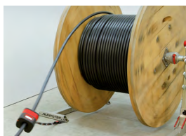
RM35 mit RUNPOLIFTER L1600 und 3 x 35 mm² Kabel
